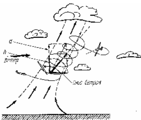
Рис 30 В ветреную погоду планер в наборе высоты сносится по ветру больше, чем восходящий поток: а — скорость ветра по ветру, б — скороподъемность планера
