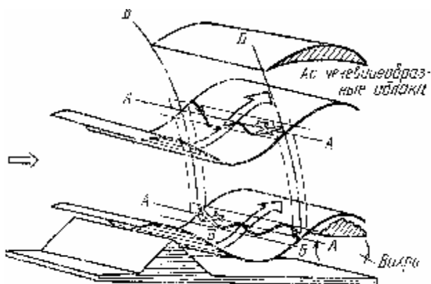
Рис. 64 Схема полета планера в области волны
