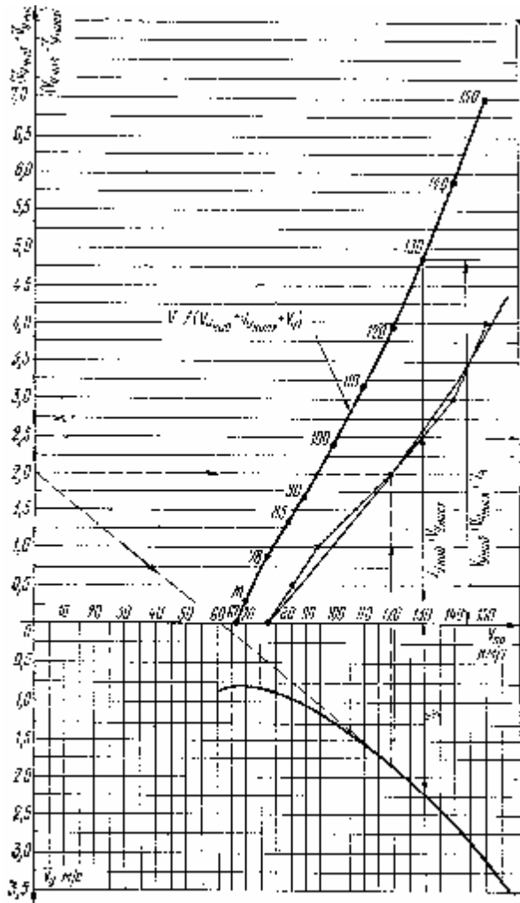
Рис. 20. Графическое определение скоростей для кругового калькулятора (Планер «Бланк», вес планера 472 кг)
