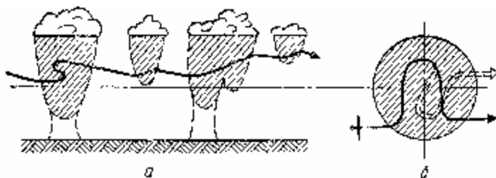
Рис. 33 а — схема движения планера «дельфин» на коротком отрезке облака под грядкой, б — S-образный маневр
