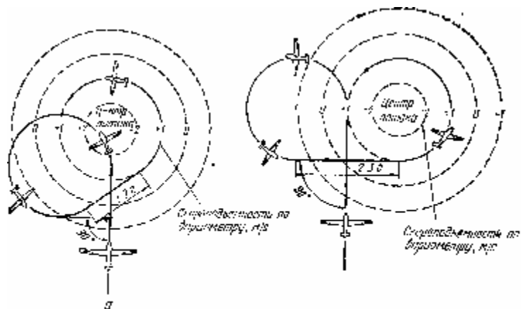
Рис 29 Центрирование планера в восходящем потоке методом вытягивания спирали а — выходящий поток вперед б — восходящий поток справа
