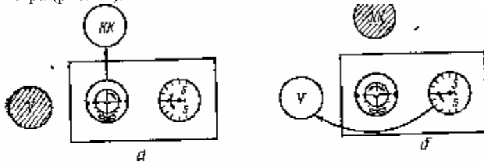
Рис 44 Последовательность переключения внимания с приборов пилотирования на приборы контроля режима полета а — отклонения по крену односторонние, в стрелок вариометра — равномерные ПРОВЕРЬ КУРС!, б — отклонения по крену равномерные, а стрелок вариометра — односторонние ПРОВЕРЬ СКОРОСТЬ!
