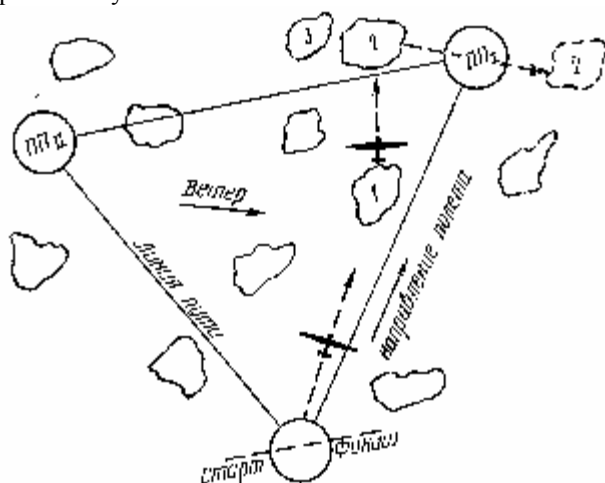
Рис 36. Один из возможных случаев отметки на поворотном пункте при полете по маршруту
