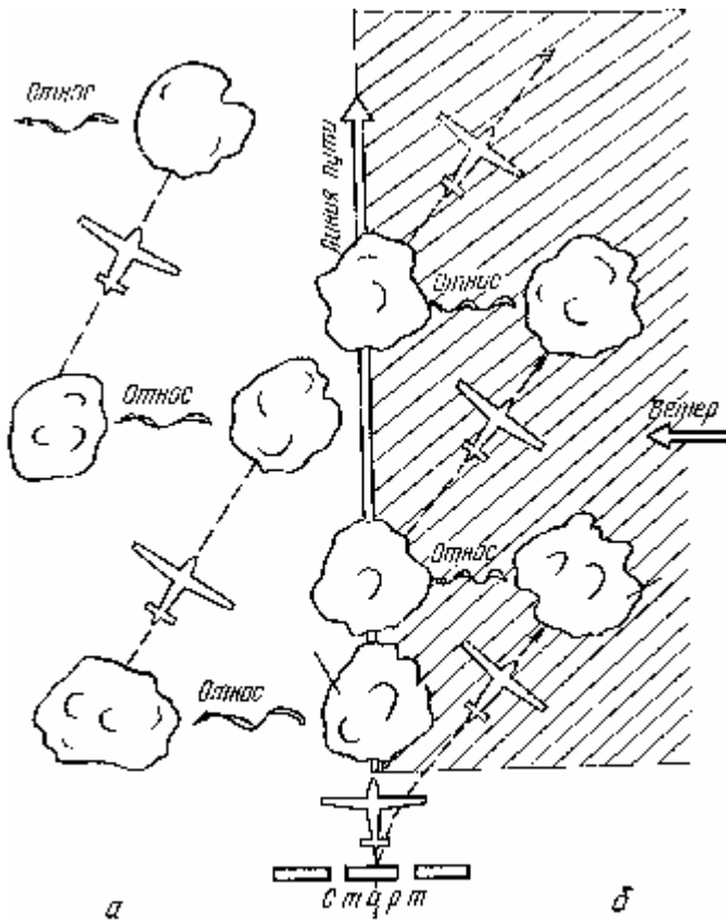
Рис. 35. Выбор направления полета после старта с учетом фактора ветра: а — неправильно; б — правильно
