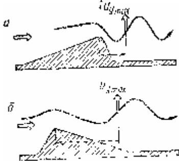
Рис 56 За асимметричными хребтами возникают подветренные волны значительной амплитуды в большем диапазоне длин волн
