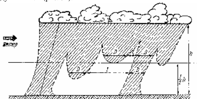
Рис. 31 Схема распределения восходящих и нисходящих потоков воздуха над грядой
