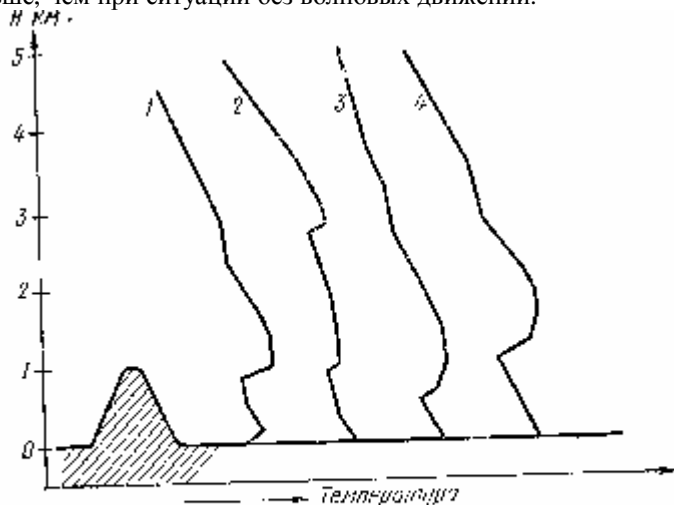
Рис 49 1, 2, 3, 4 — характерные кривые стратификации атмосферы, при которых возникают волновые движения над препятствиями
