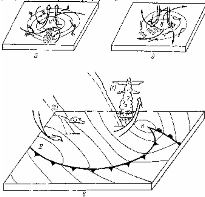
Рис. 7. Основные барические системы: а — сходимость воздушных течений в циклоне, б — расходимость воздушных течений в антициклоне, в — циклонический (1) и антициклонический (2) типы фронтов
