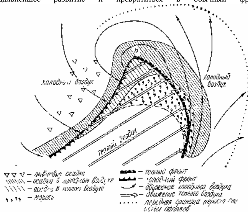
Рис 9 Модель циклонического вихря
