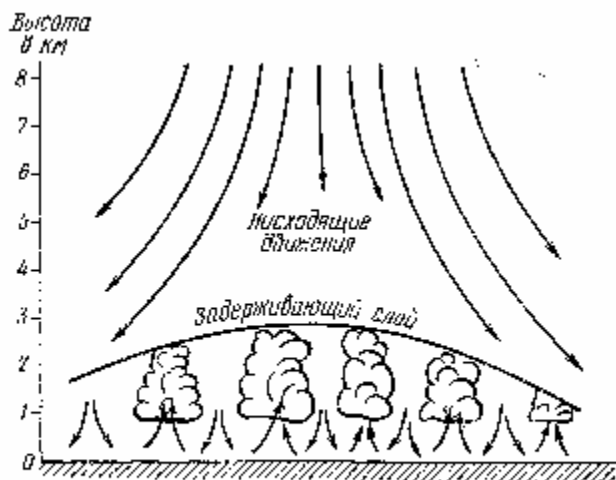
Рис 8 Схематическое изображение погоды в ядре антициклона
