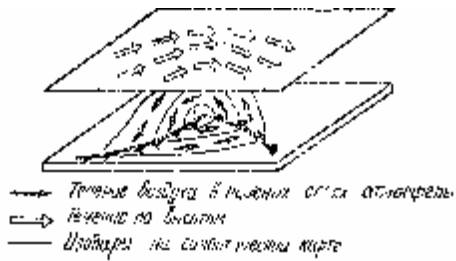
Рис. 54 Синоптческая обстановка, при которой направление и скорость ветра по высотам наиболее благоприятны для образования волновых движений
