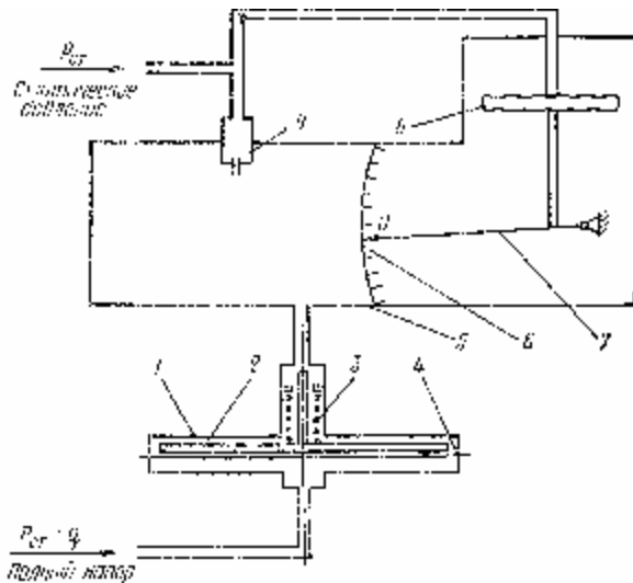
Рис. 24. Обобщенная схема вариометра с компенсатором: 1 — корпус регулятора (компенсатора); 2 — поршень регулятора с пружиной 3; 4 — капилляр регулятора с жесткостью K ; 5 — камера регулятора с жесткостью K ; 6 — мембрана из тонкой эластичной резины, исключившая перетекание воздуха между полостями регулятора; 7 — корпус вариометра; 8 — шкала; 9 — стрелка; 10 — мембрана; 11 — капилляр; 12 — камера.
