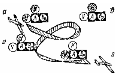
Рис. 46. Распределение внимания на приборы при выполнении спирали: а — вход в спираль; б — устойчивая спираль (вторая половина); в — устойчивая спираль (первая половина); г — выход из спирали
