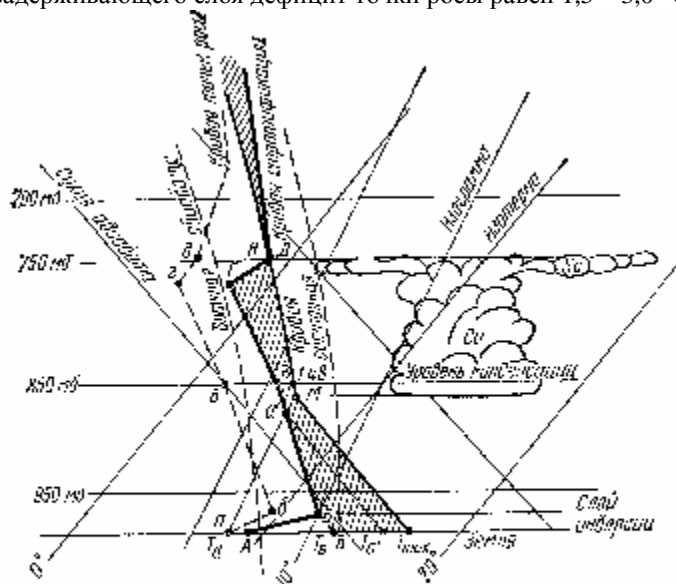
Рис. 15 Наличие задерживающего слоя выше уровня конденсации (в данном случае участок ГД на кривой стратификации) и увеличение влажности с высотой вызывает растекание кучевой облачности Си в 8—10-балльную слоисто-кучевую Sc
