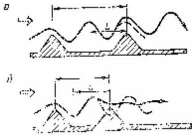
Рис. 57 Влияние двух горных хребтов, расположенных последовательно друг за другом, на интенсивность вынужденного движения
