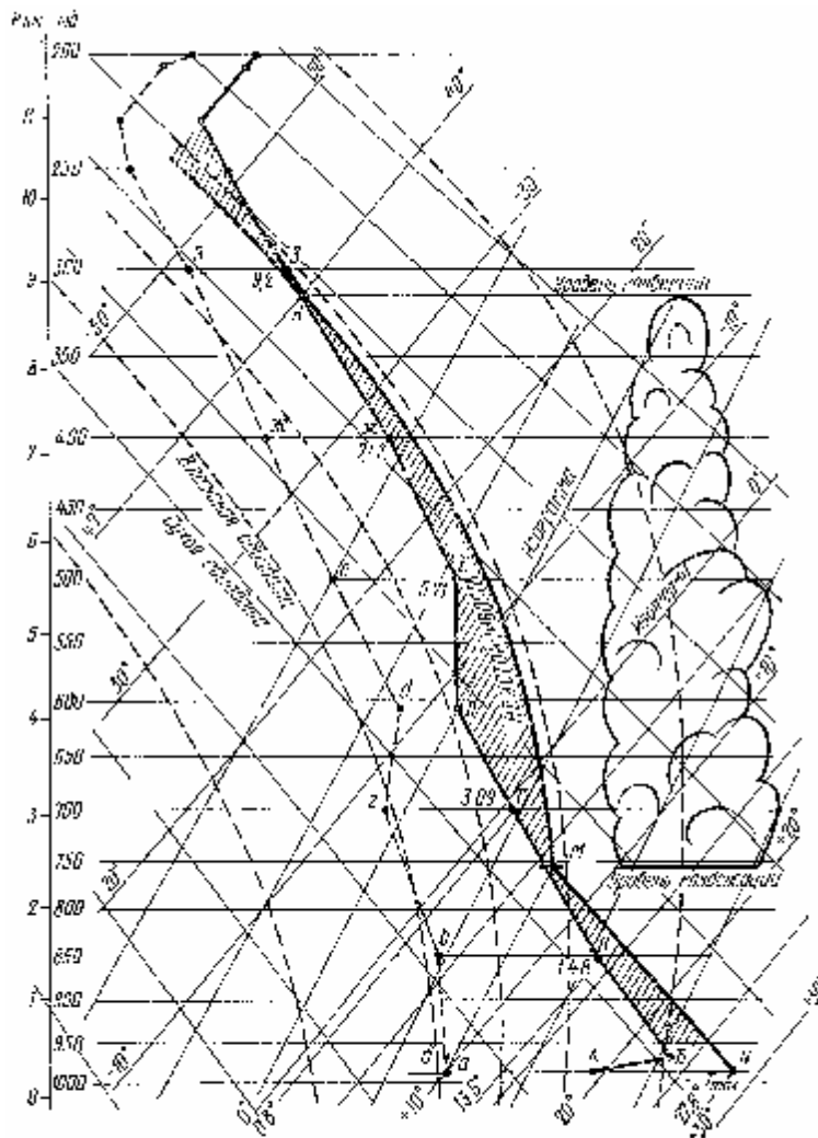
Рис 13 Пример построения кривых стратификации, точек росы и состояния по данным радиозондирования атмосферы: АВВГДЕЖЗ — кривая стратификации; абвгдежаз — кривая точек росы, АМП — кривая состояния
