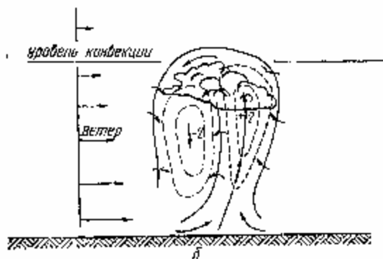
Рис. 27 Скор потока и характер вертикальных потоков под облаками при палочке пескыного ветра а — усиливающегося с высотой, б — слабеющего с высотой
