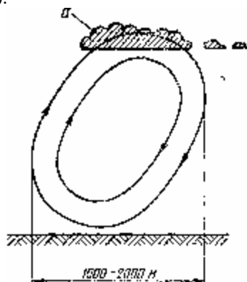
Рис. 61. Вертикальный разрез обычно встречаемого ротора (вихря) (а — разорвавшиеся роторные облака)
