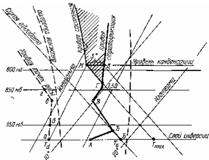
Рис 14 В данном примере аэрологическая диаграмма указывает на то, что выше 1500 м «термики» распространяться не будут, так как вклетке атмосфера стратифицирована устойчиво (кривая состояния расположена левее кривой стратификации). В течение дня ожидается ясная безоблачная погода, точка M лежит левее кривой стратификации при 3^{\circ}\text{C} .
