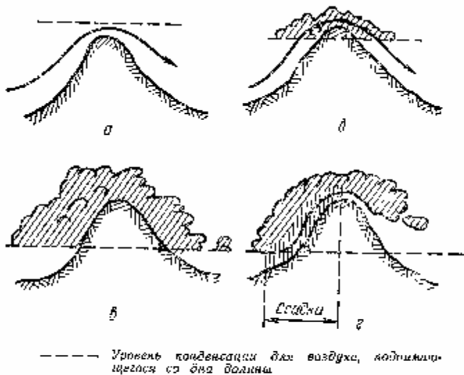
Рис 59 Различные случаи образования вала облаков фенового ветра при условии, что уровни долин, окружающих горный хребет, с обеих сторон одинаковы
