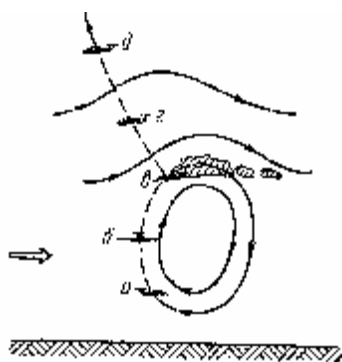
Рис 67 Переход из роторных движений на волновые в случае относительно слабого ветра
