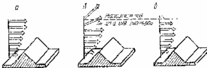
Рис. 53 Скорость и направление ветра по высоте существенно зависит на ристроостранстве и образующие волнового движения в атмосфере
