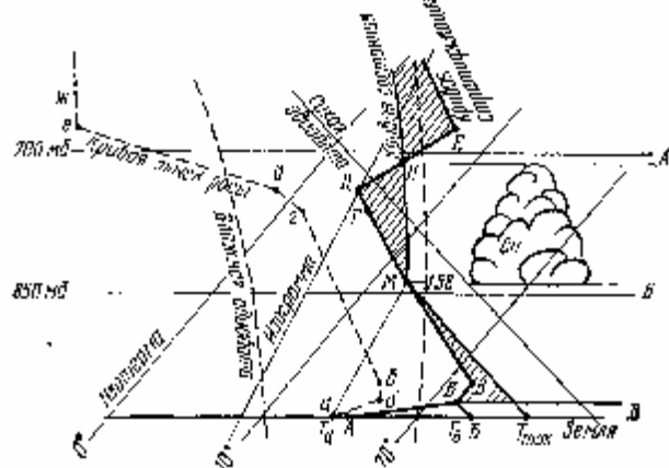
Рис. 16 Если на нижней границе задерживающего слоя (в данном примере на кривой стратификации слой ДЕ) дефицит точки росы равен или более 5° С, то с верхней границы облаков происходит интенсивное испарение. Растекания кучевых облаков не происходит
