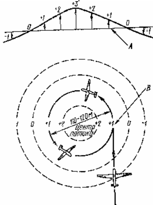
Рис. 28 Один из примеров входа планера в восходящий поток и рис. предельные скороподъемности по диаметру потока
